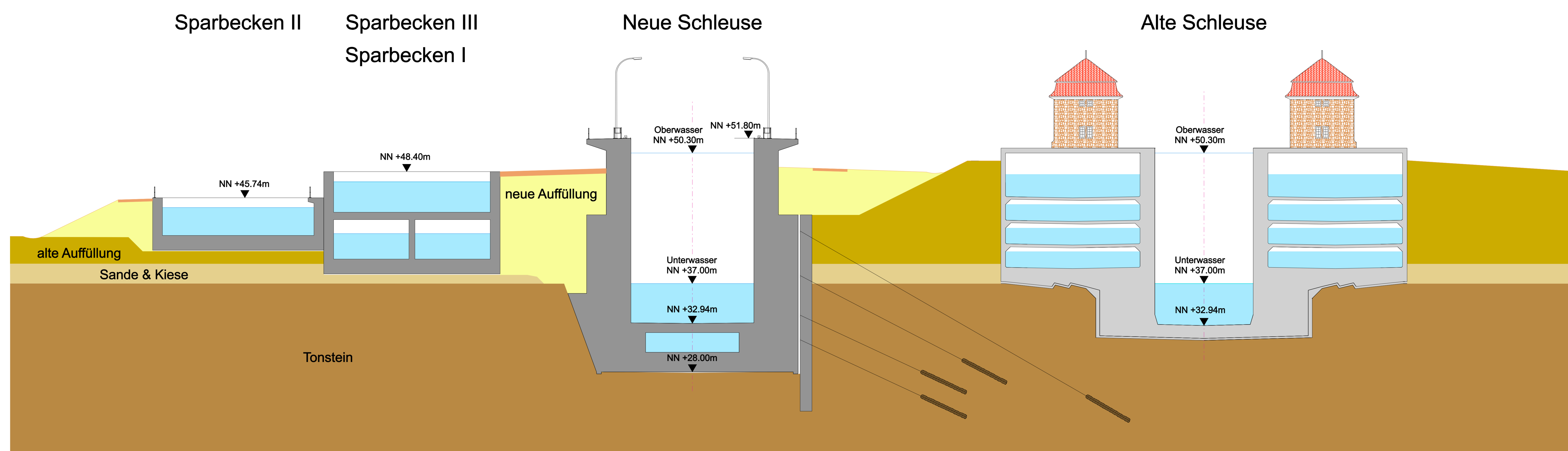
Querschnitt
